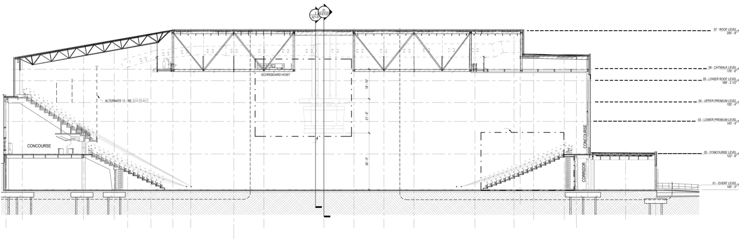
LONGITUDINAL SECTION 5/16" = 1' - 0"
